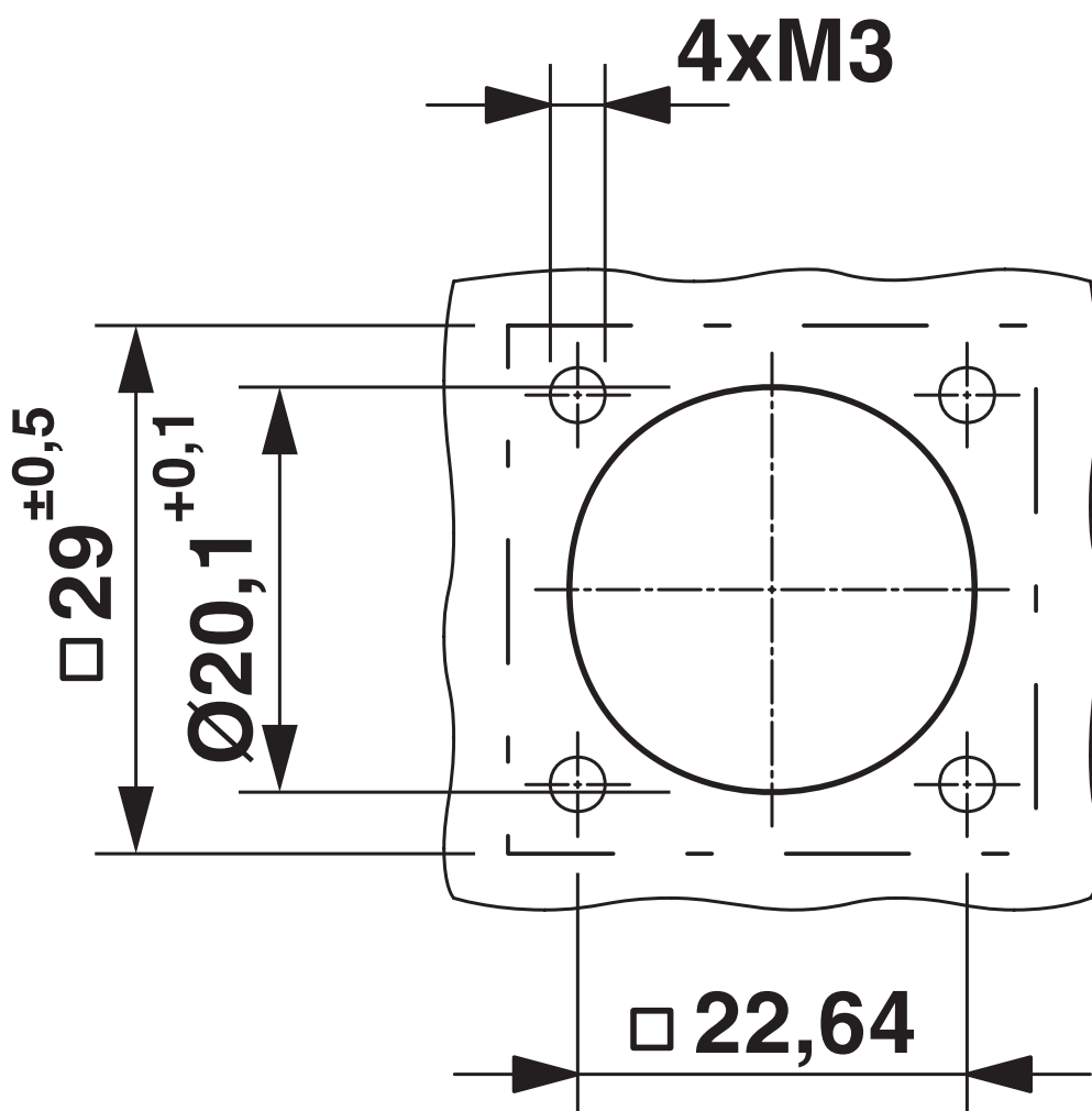
Rysunek wymiarowy
