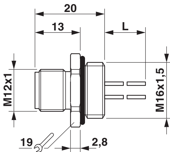
Rysunek wymiarowy
