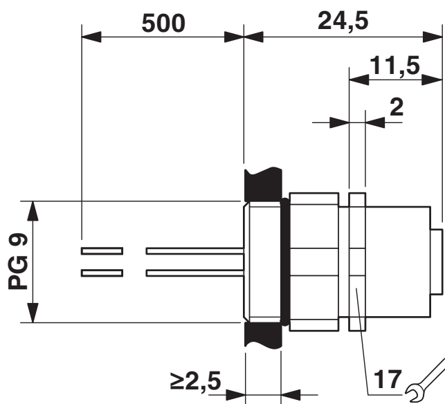
Rysunek wymiarowy
