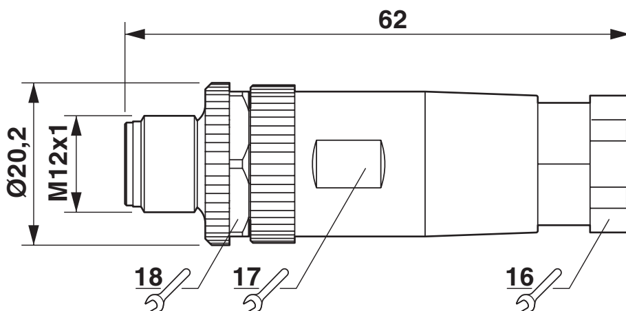
Rysunek wymiarowy
