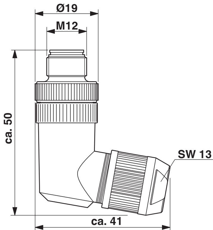
Rysunek wymiarowy
