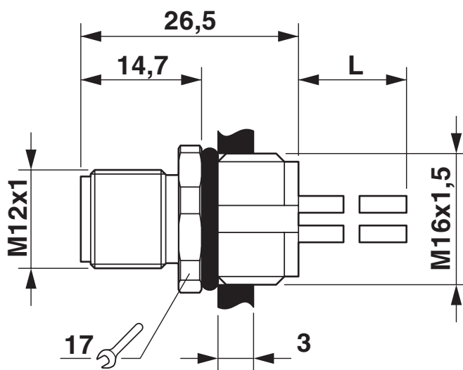
Rysunek wymiarowy
