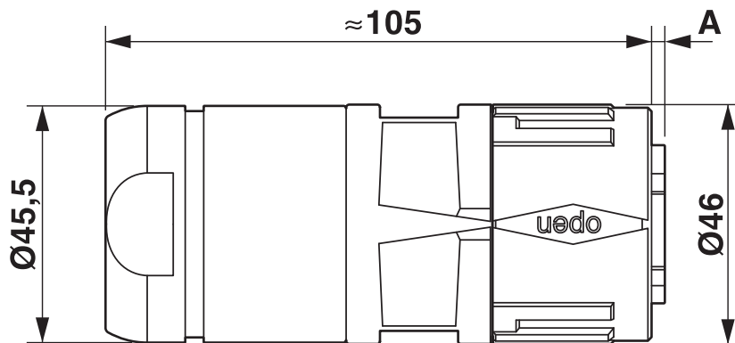
Rysunek wymiarowy
