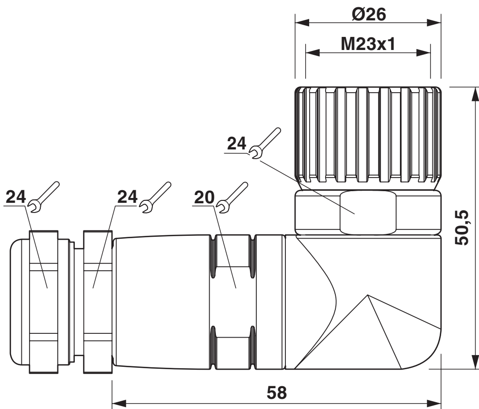
Rysunek wymiarowy
