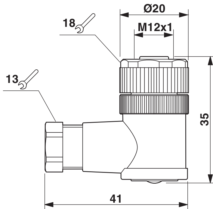
Rysunek wymiarowy
