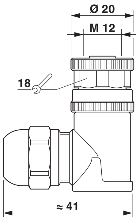
Rysunek wymiarowy
