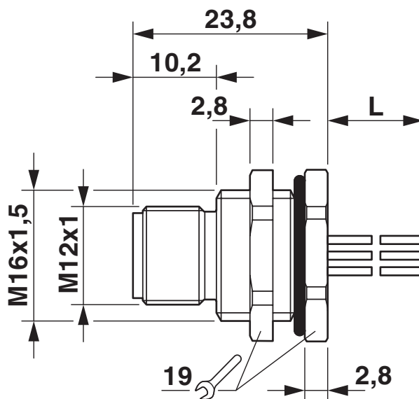
Rysunek wymiarowy
