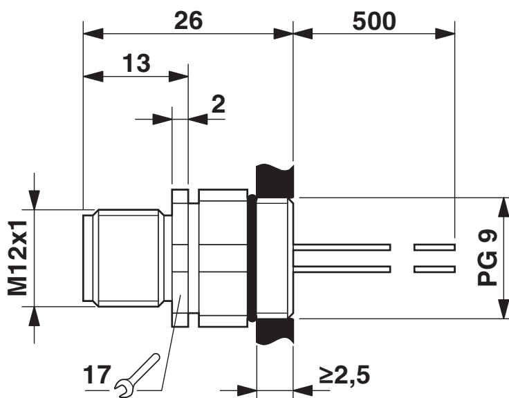
Rysunek wymiarowy
