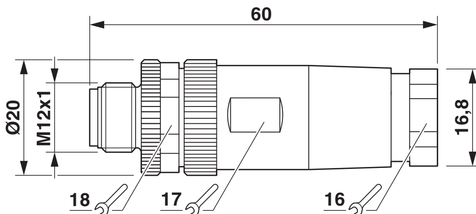
Rysunek wymiarowy
