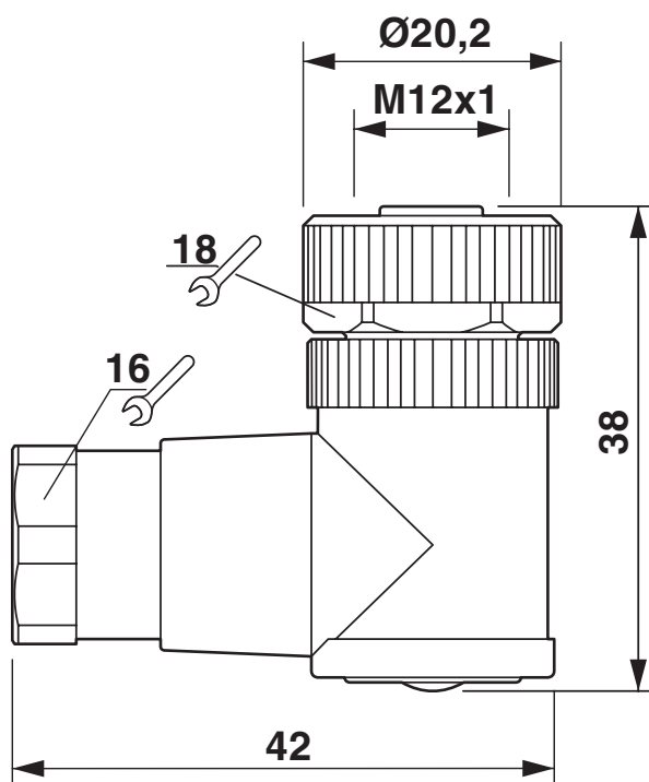
Rysunek wymiarowy
