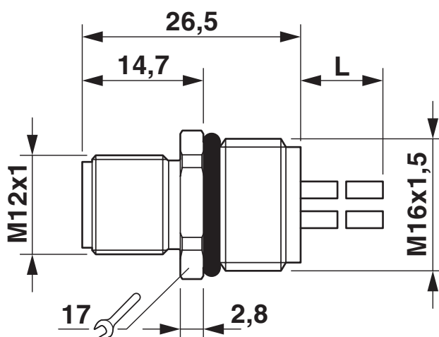
Rysunek wymiarowy
