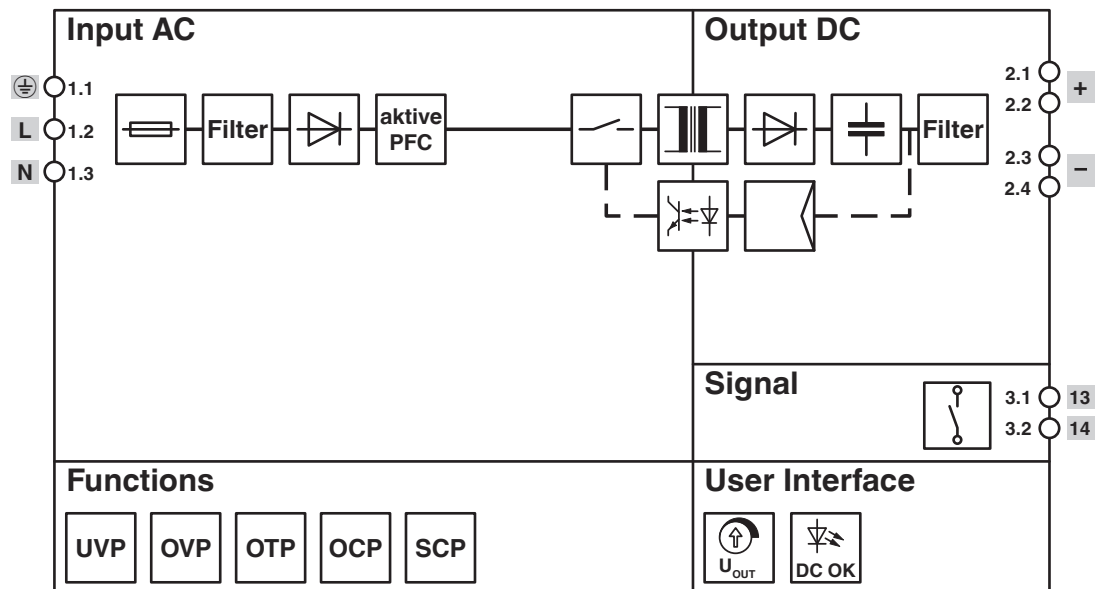
Schemat blokowy
