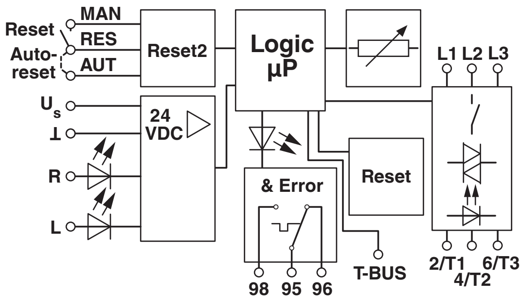
Schemat blokowy
