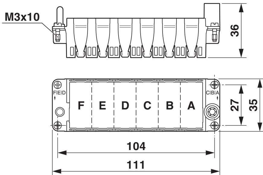
Rysunek wymiarowy
