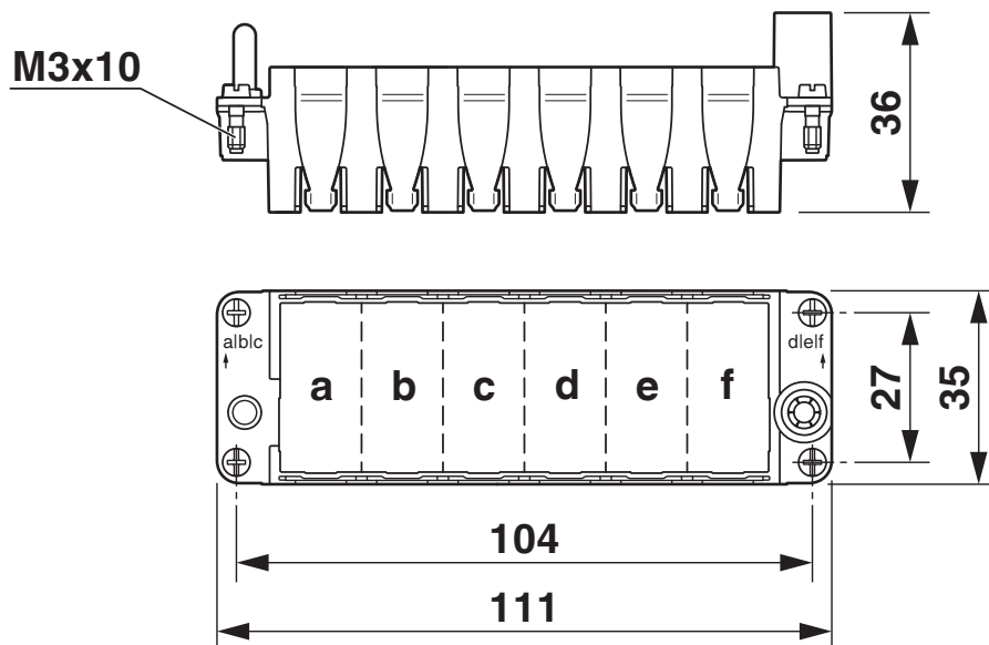
Rysunek wymiarowy
