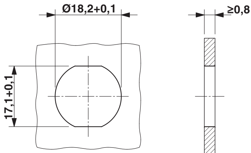
Rysunek wymiarowy
