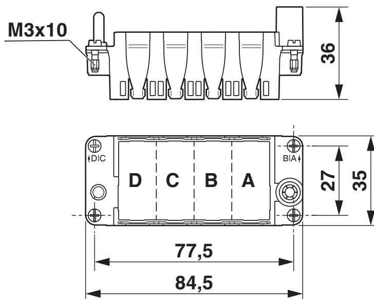
Rysunek wymiarowy
