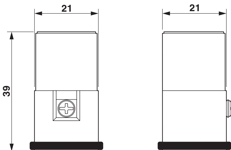
Rysunek wymiarowy
