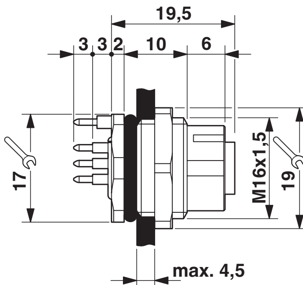
Rysunek wymiarowy
