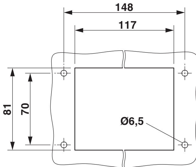
Rysunek wymiarowy
