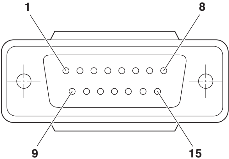
Schemat
