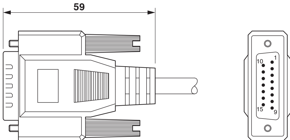
Rysunek wymiarowy
