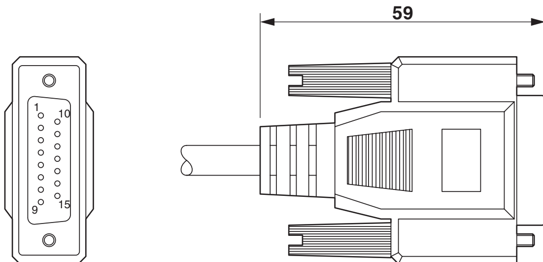
Rysunek wymiarowy
