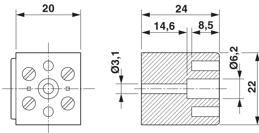
Rysunek wymiarowy
