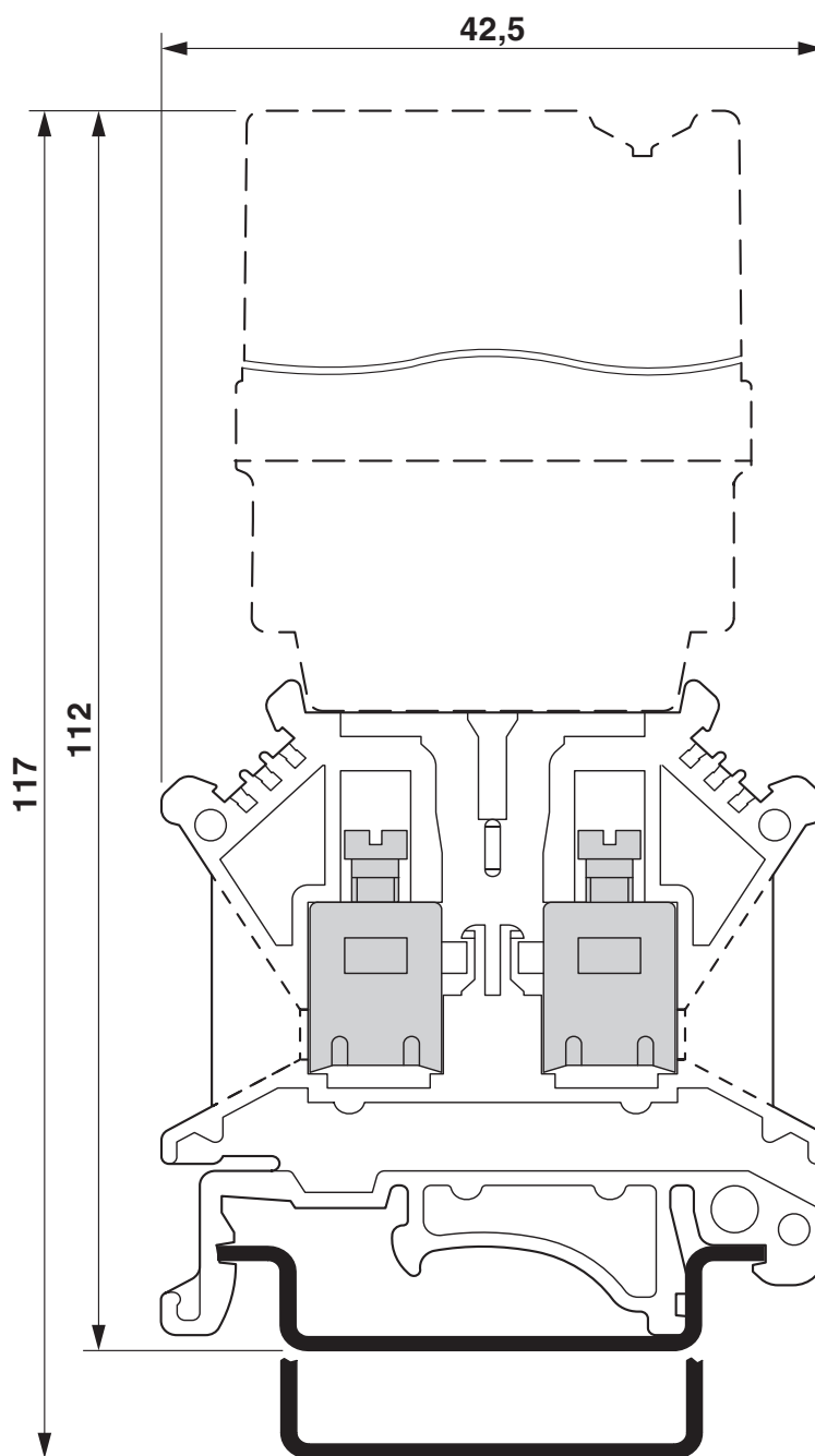
Rysunek wymiarowy
