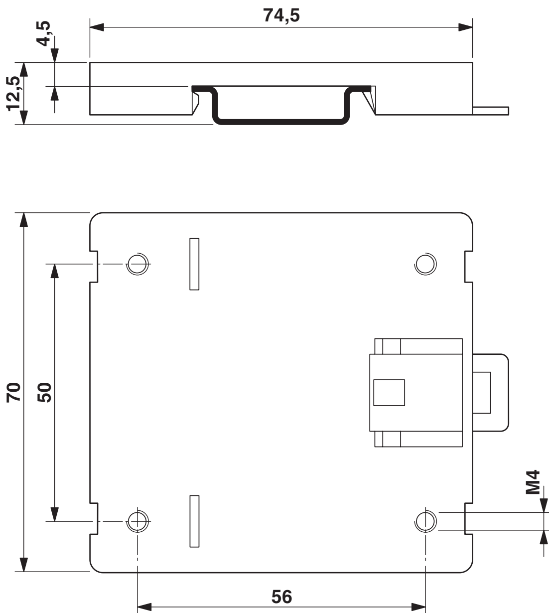
Rysunek wymiarowy
