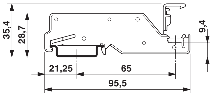
Rysunek wymiarowy
