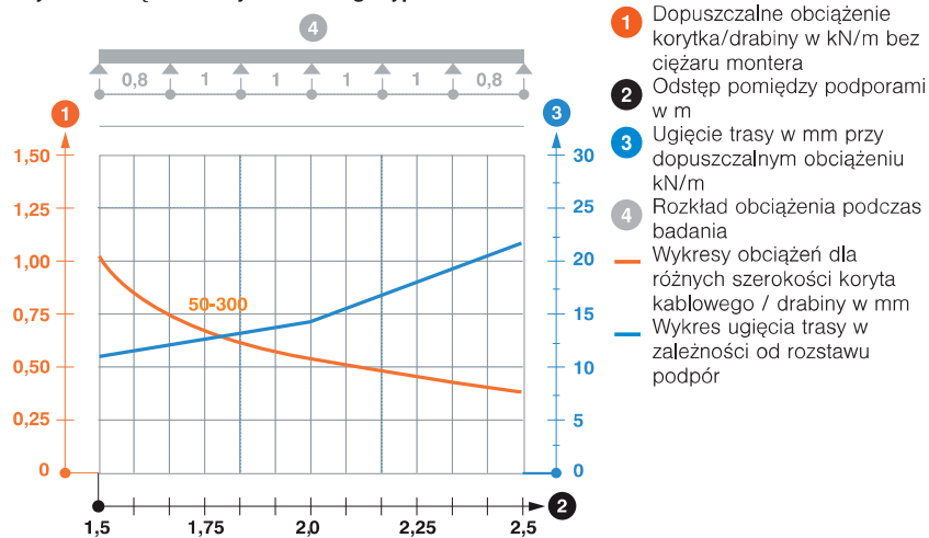
Wykres obciążenia koryta kablowego typ RKS 35
