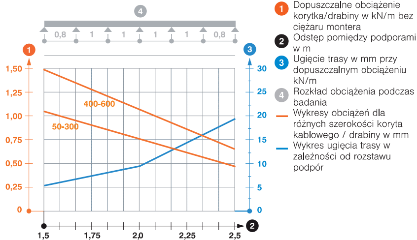
Wykres obciążenia koryta kablowego typu RKS 60
