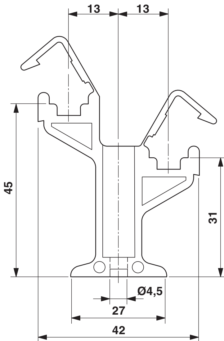
Rysunek wymiarowy
