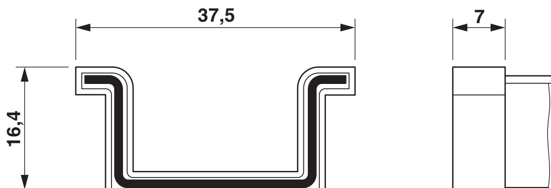
Rysunek wymiarowy
