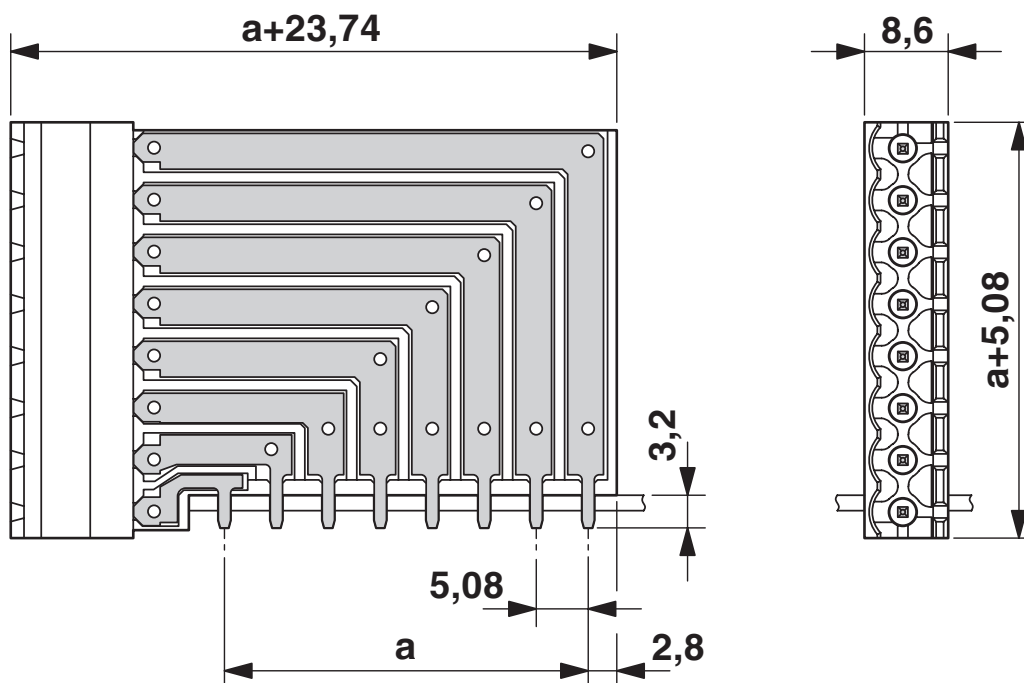
Rysunek wymiarowy
