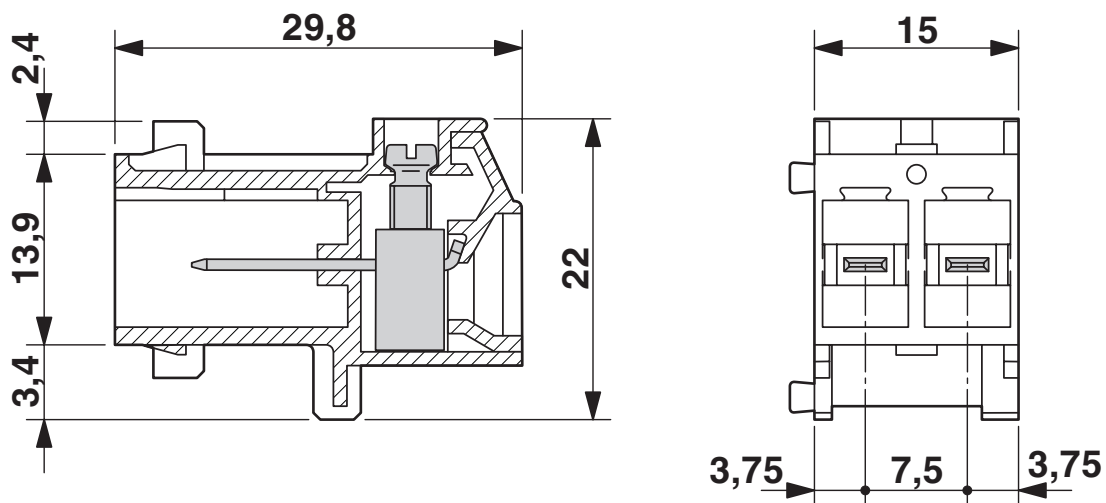
Rysunek wymiarowy
