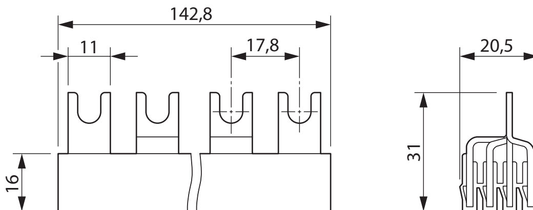
Rysunek wymiarowy
