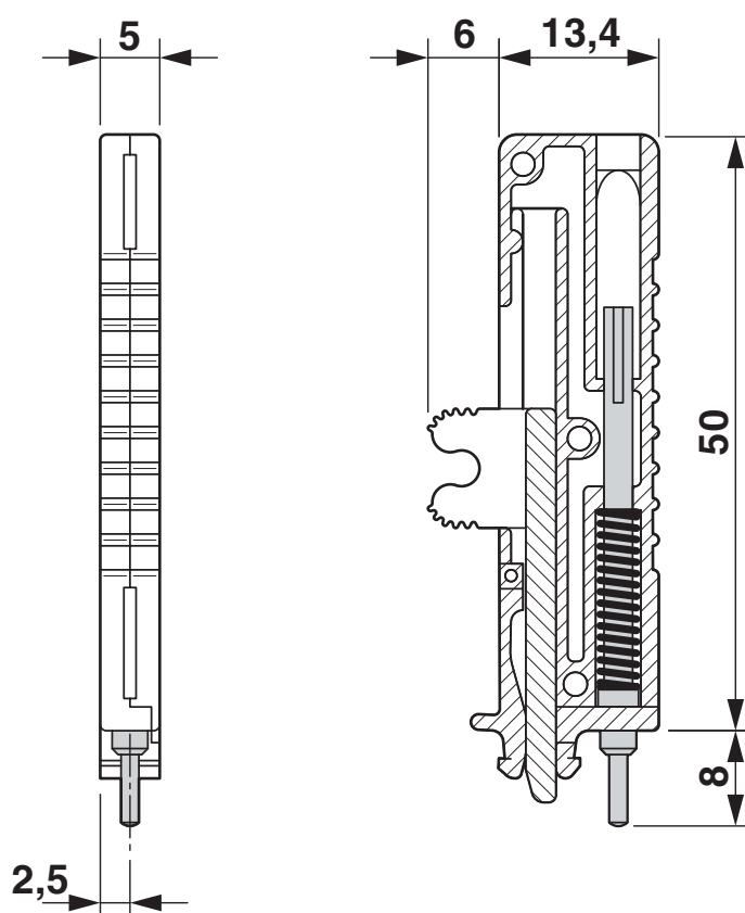
Rysunek wymiarowy
