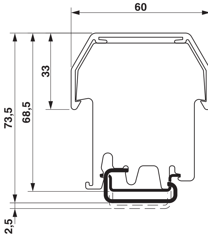
Rysunek wymiarowy
