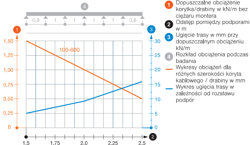
Wykres obciążenia koryta kablowego typ MKS 60
