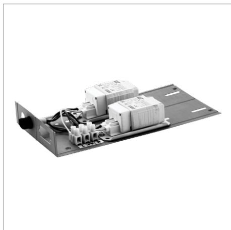
płyta montażowa
