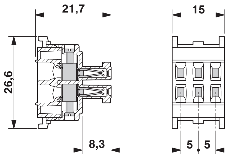
Rysunek wymiarowy
