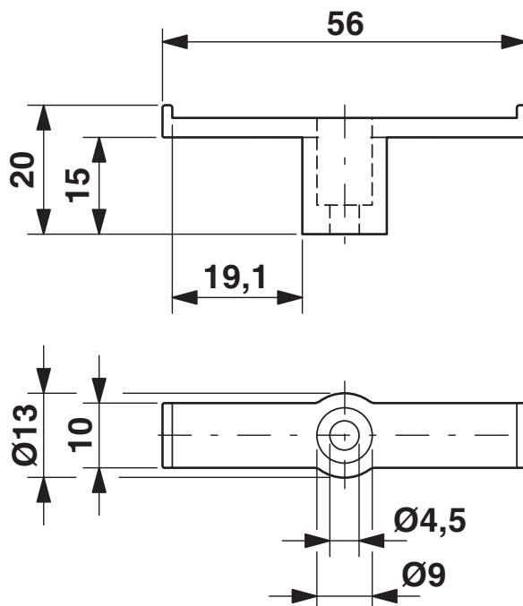
Rysunek wymiarowy
