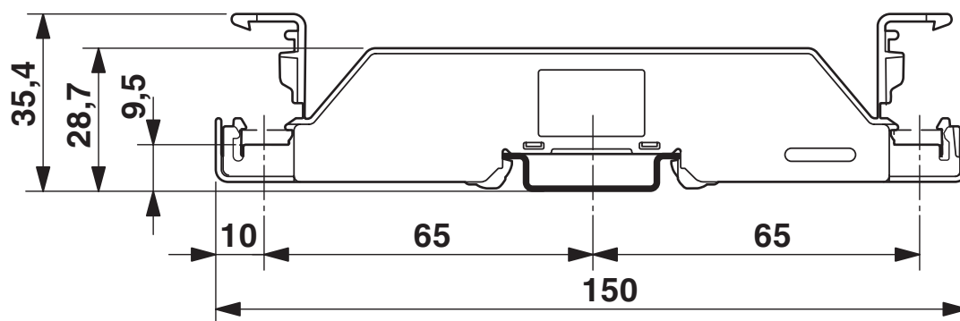
Rysunek wymiarowy
