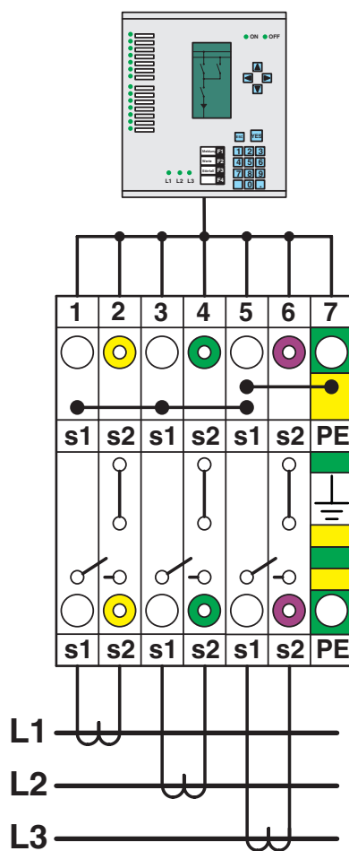
Rysunek schematyczny
