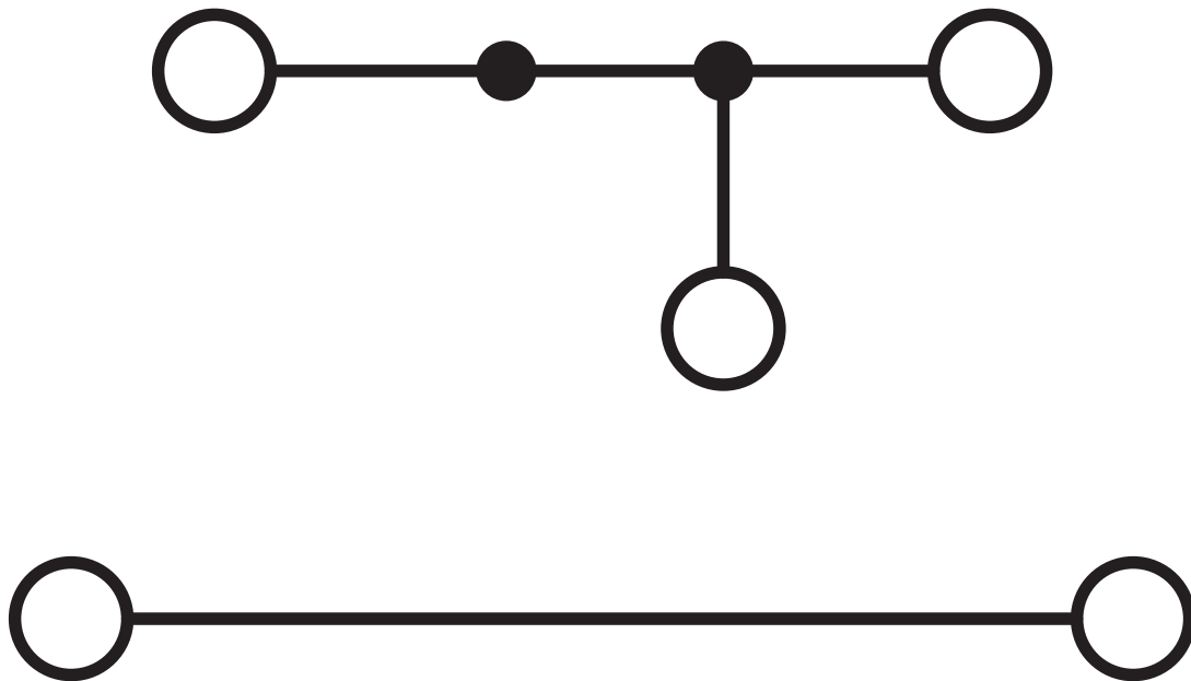
Schemat
