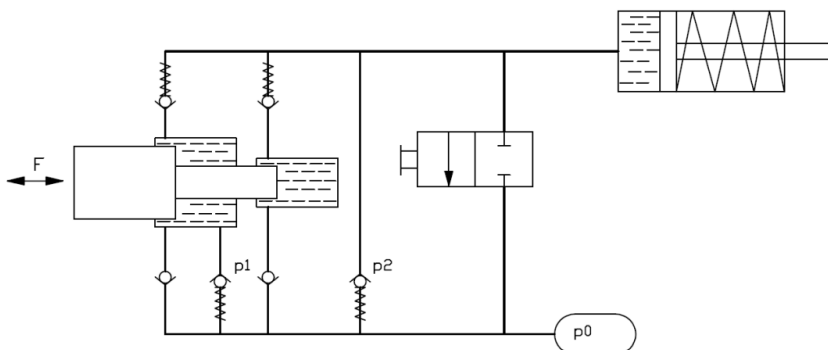
Rys. 4. Schemat hydrauliczny.
