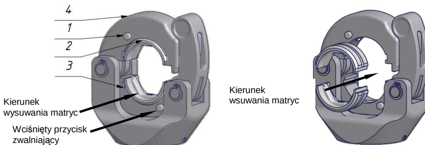
Rys. 1. Zmiana matryc.
