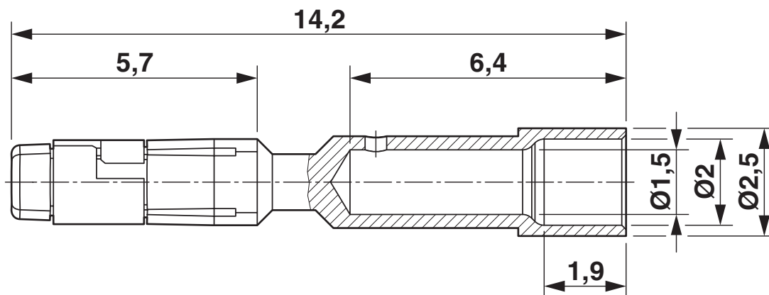
Rysunek wymiarowy
