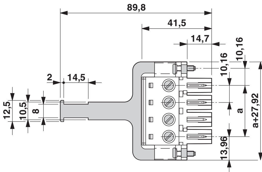
Rysunek wymiarowy
