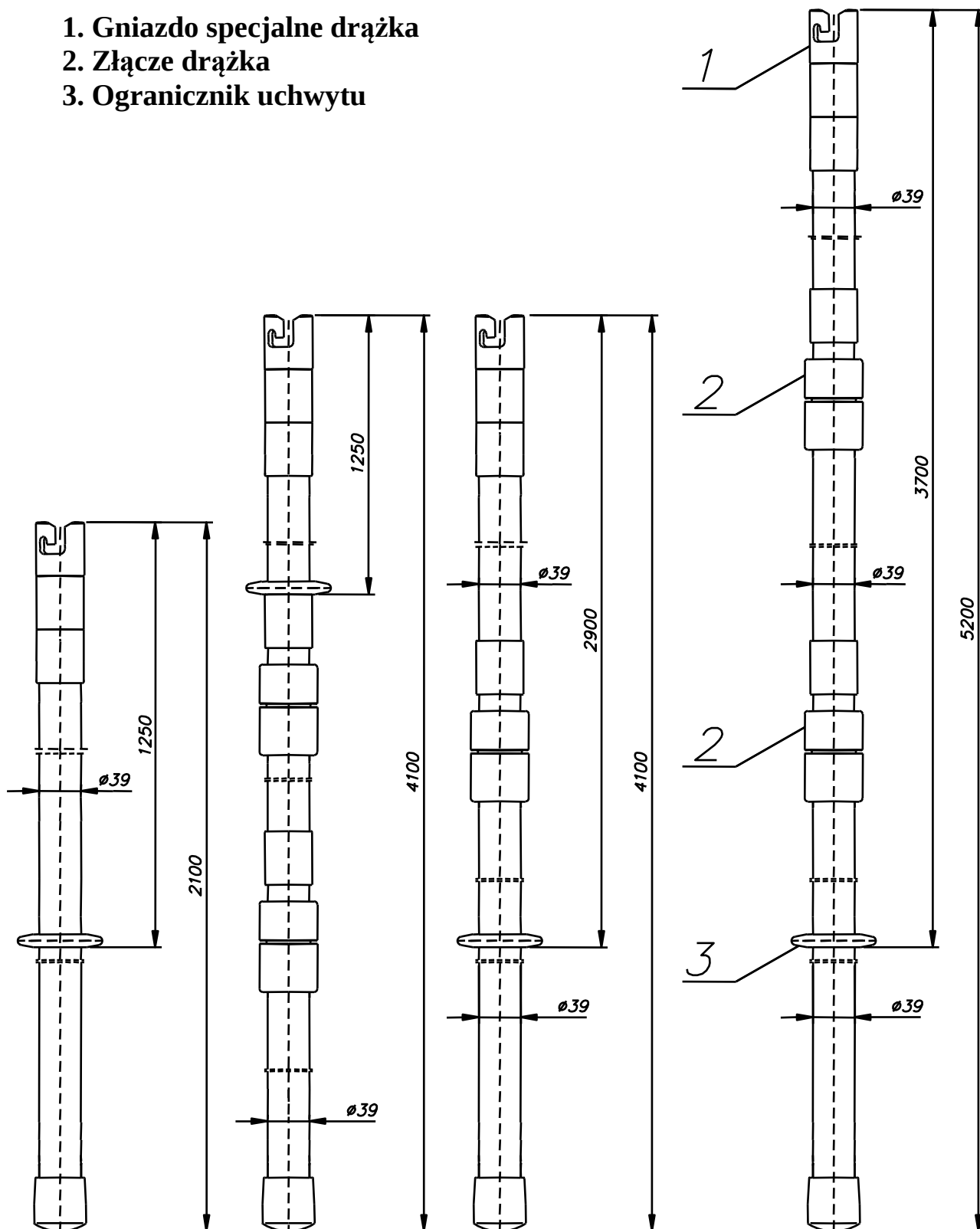
Drażek DIPS-110-B
