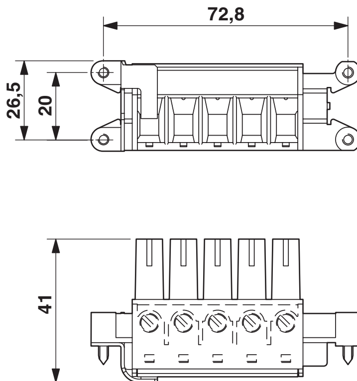
Rysunek wymiarowy
